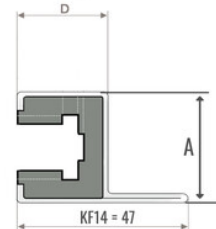
Guide en "KF" monté sur rail 14 "KF" guide with 14
