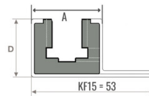
Guide en "KF" monté sur rail 15 "KF" guide with 15
