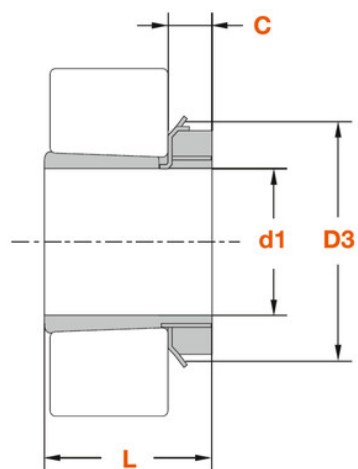
Manchon de serrage
