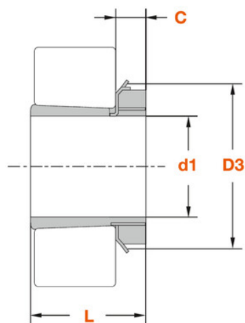
Manchon de serrage
