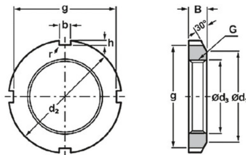
Ecou monté avec rondelle de blocage séries AN05/KM05 à AN40/KM40
